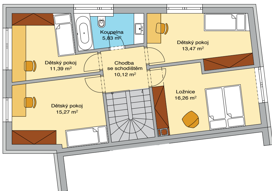
Půdorys 2.NP
