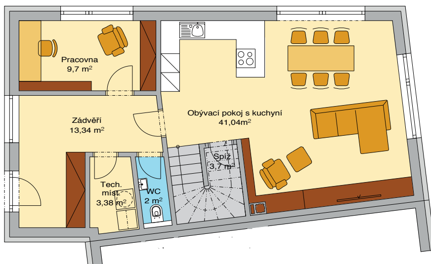
Půdorys 1.NP
