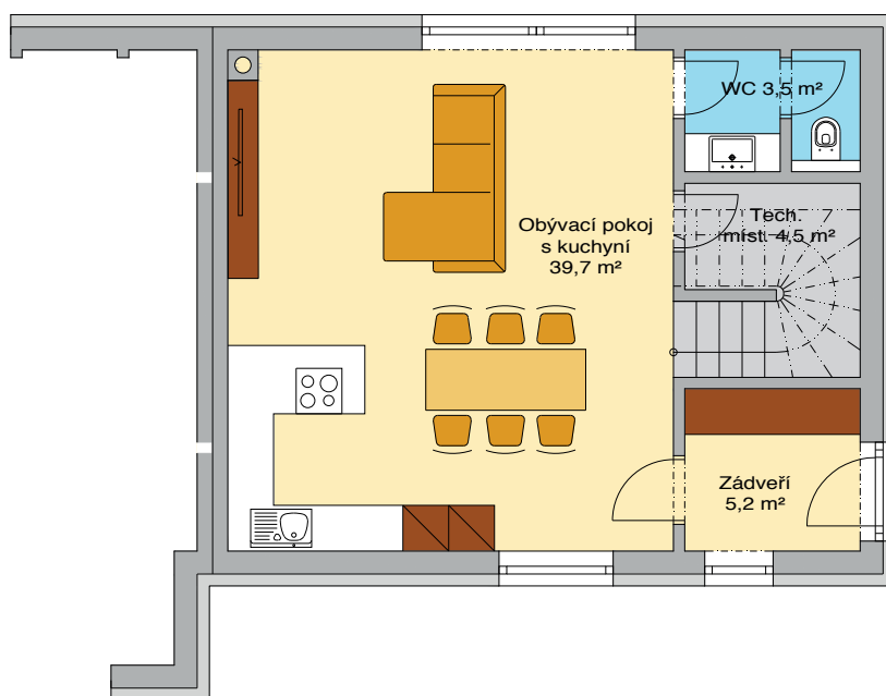
Půdorys 1.NP
